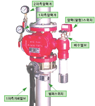
▲ 알람밸브의 구성 및 명칭
